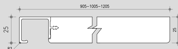
Sezione anta orizzontale Horizontal door section
