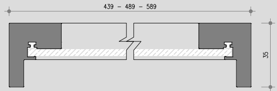
Sezione anta orizzontale Horizontal door section
